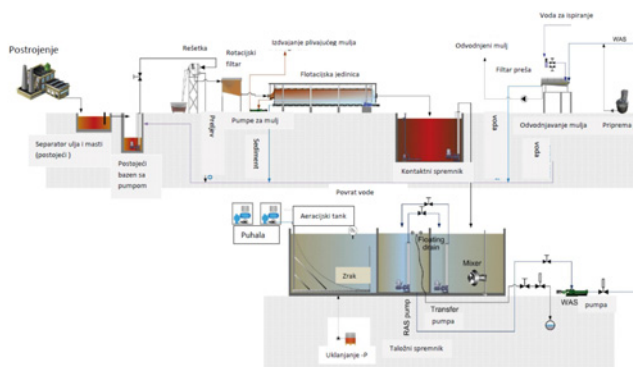
Slika 1. Tehnološka shema sustava za pročišćavanje otpadnih voda
